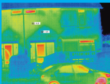
Detectie van uitgezakte isolatie in een spouwmuur
