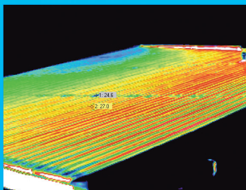
Thermische opname van een dak met vochtproblemen
